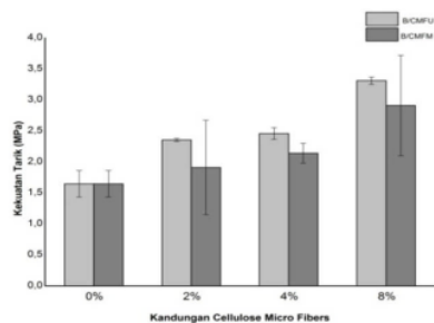
Gambar 2. Kurva kekuatan tarik komposit bioplastik.
