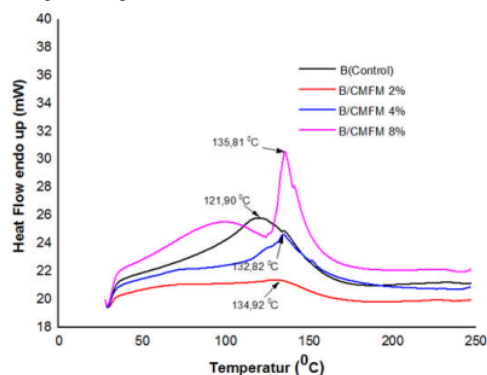
Gambar 5. Grafik DSC komposit bioplastik dengan perbedaan konsentrasi filler CMFM .
