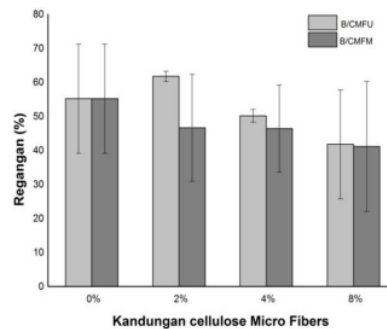
Gambar 3. Kurva regangan komposit bioplastik.
